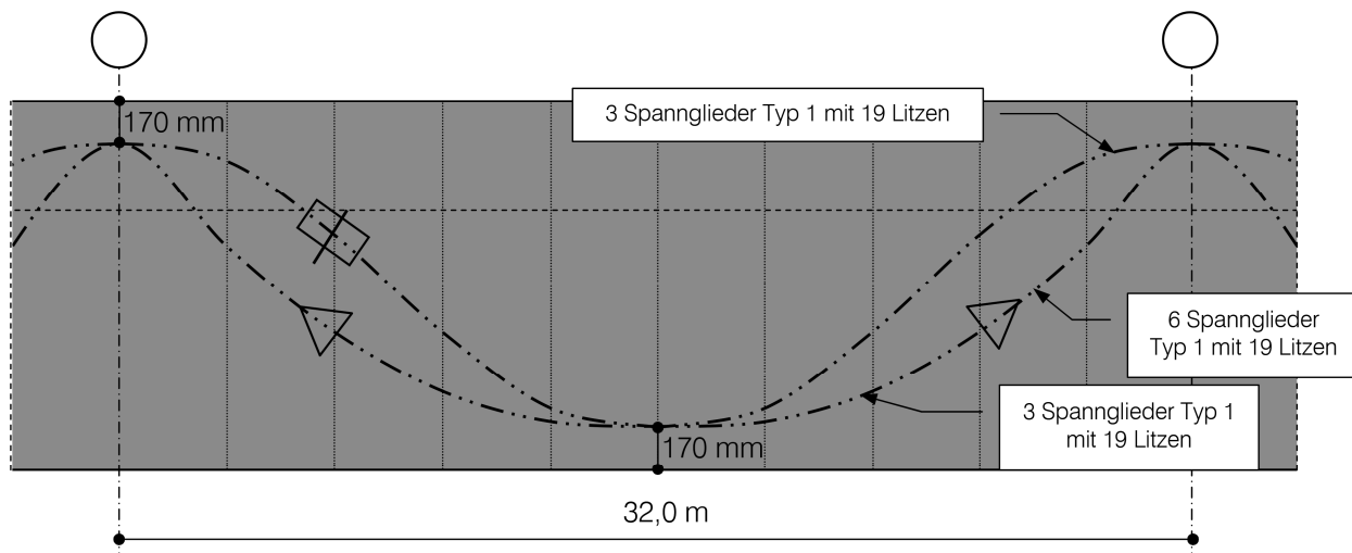
Bild 5: Spanngliederverlauf im Aufriss (schematisch für das Innenfeld)
