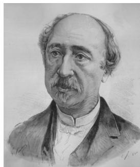
E. Becquerel (1820–1891)
