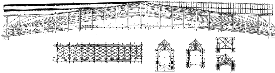
Abb. 1.4 Entwurf einer Brücke über den Rhein bei Schaffhausen, Grubenmann , 1755.
