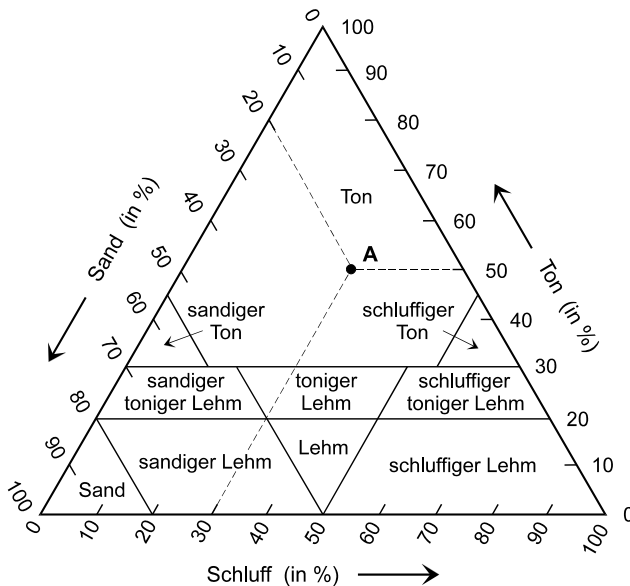
Bild 1-10 Dreiecknetz der Public Roads Administration zur Bodenklassifizierung (nach Terzaghi [250])
