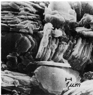
a) Kaolin
