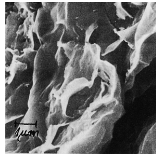
c) Montmorillonit
