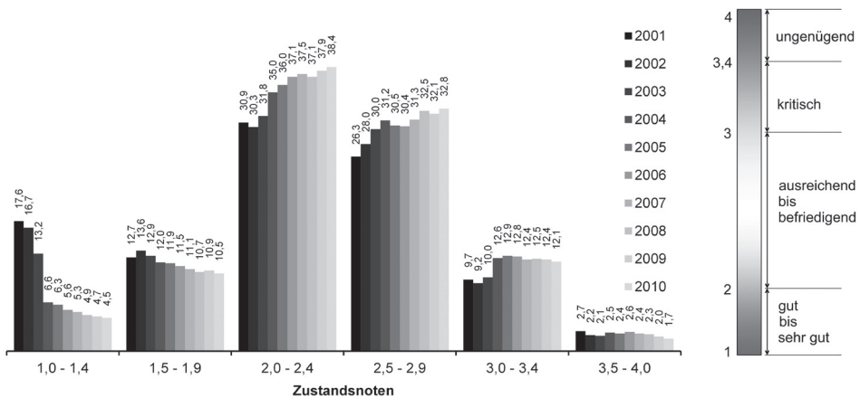
Bild 6. Entwicklung der Zustandsnoten für Brücken an Bundesfernstraßen mit Bewertung nach RI-EBW-PRÜF (nach [18, 19])
