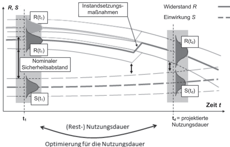
Bild 19. Entwicklung von Tragwiderstand R und Einwirkung S über die Zeit [76]
