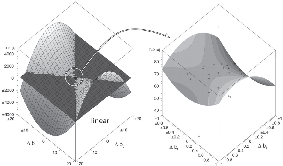
Bild 23. Zweiparametrische Antwortfläche mit Detailausschnitt
