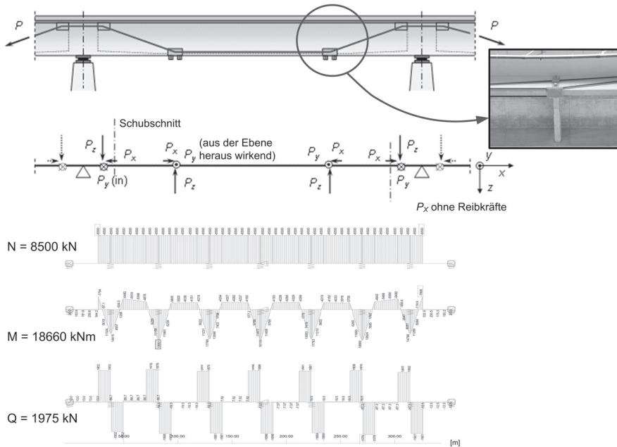
Bild 18. Verstärkung mit umgelenkten externen Spanngliedern und zugehörige Schnittgrößenverläufe (nach [69])
