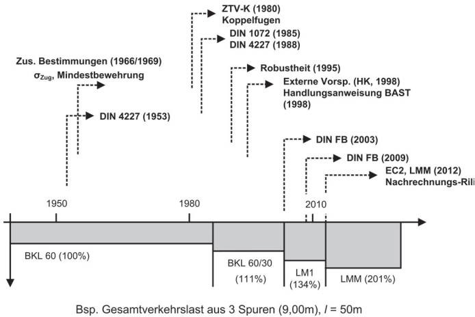
Bild 8. Ausgewählte Entwicklungsschritte der Verkehrslasten, Vorschriften und technischen Neuerungen für Spannbetonbrücken über die vergangenen Jahrzehnte
