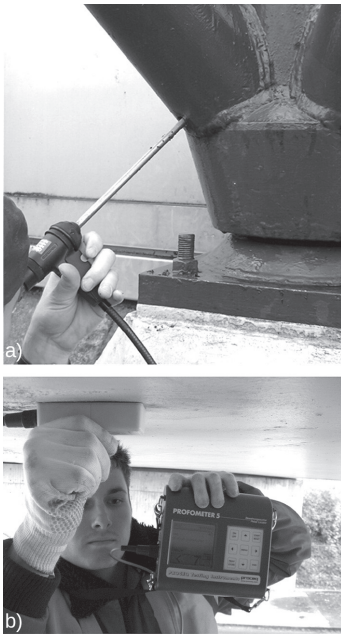
Bild 11. a) Endoskopische Untersuchung, b) Messung der Betondeckung (nach [13])
