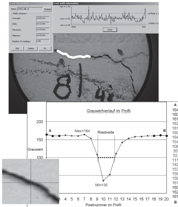
Bild 13. Aufnahmebereich und Auswertungsdiagramm einer Risskamera (nach [30])
