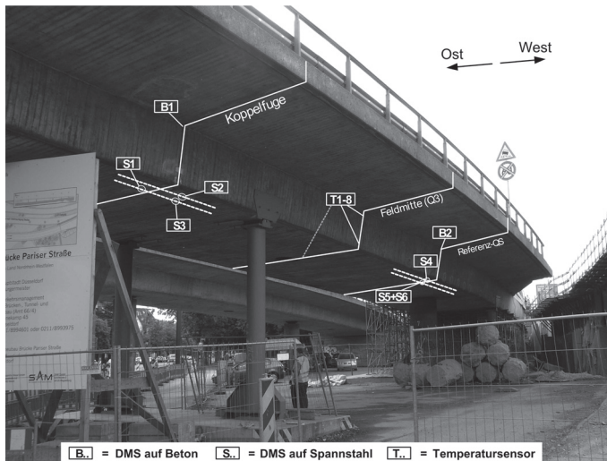
Bild 15. Messquerschnitte an der Brücke „Pariser Straße“ in Düsseldorf
