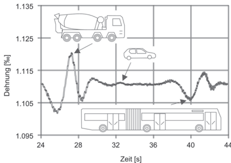
Bild 16. Videoabgleich von Verkehrseinwirkungen mit den Messwerten von Dehnungsmessstreifen [45]
