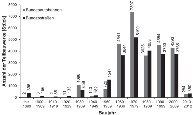
Bild 2. Altersstrukturen der Straßenbrücken im Zuge der Bundesfernstraßen (nach [12])
