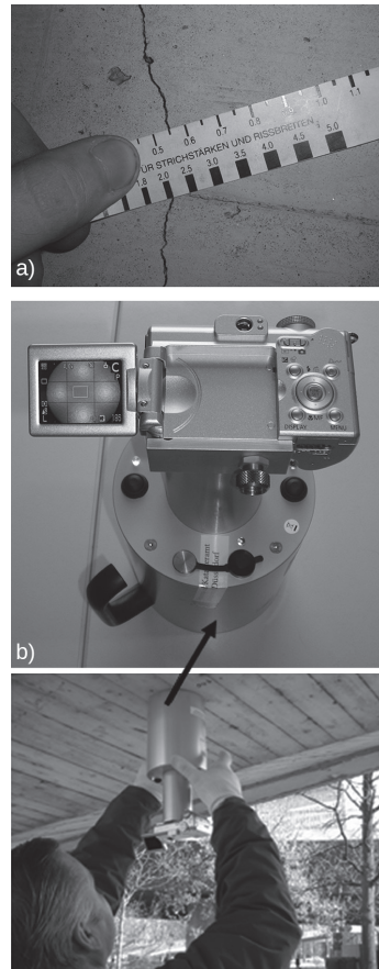
Bild 12. Rissweitenmessung mithilfe a) einer klassischen Risskarte und b) einer Risskamera [30]
