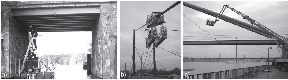
Bild 10. Hilfsgerätschaften zur handnahen Brückenprüfung; a) Leiter und Schwimmponton, b) Kabelbefahrergerät [25], c) Hubsteiger
