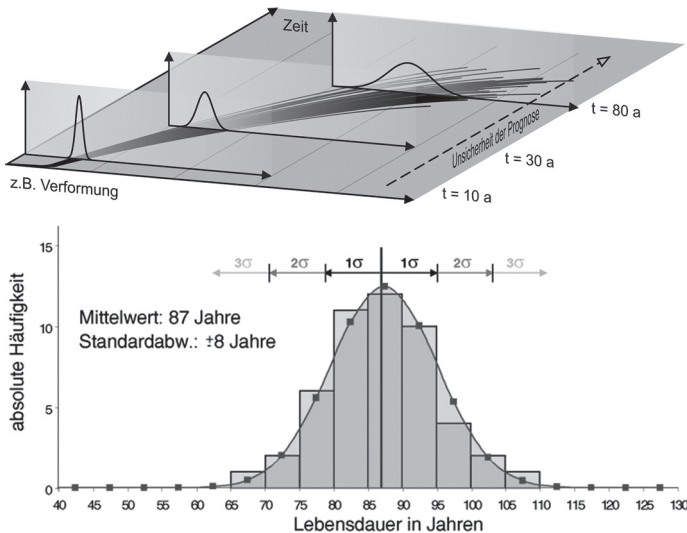
Bild 20. Entwicklung einer rechnerischen Brückenverformung über die Zeit mit Häufigkeitsverteilung einer rechnerischen Lebensdauer (vgl. [76])
