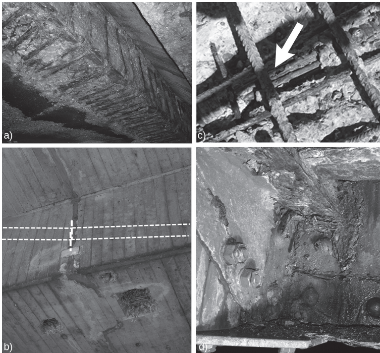
Bild 4. a) Starke Korrosionsschäden an Bewehrungsstählen eines Unterzugs, b) Risssschaden an einer Koppelfuge, eingezeichnet sind der Spanngliedverlauf sowie die Koppelstellen, c) Korrosionsschäden an internen Spanngliedern, d) Blattkorrosion an einer Stahlbrücke (nach [13])
