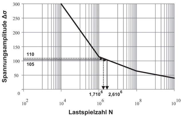
Bild 14. Beispiel zum Einfluss von Änderungen in der Spannungsamplitude auf eine Lastspielzahl
