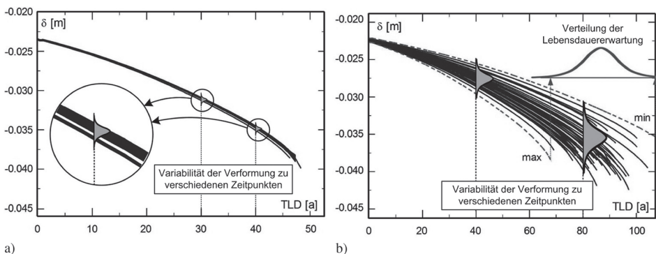
Bild 21. Aufweitung der rechnerischen Nutzungsdauer (TLD) am Beispiel a) der Betondruckfestigkeit und b) der Korrosionsrate (aus [76])
