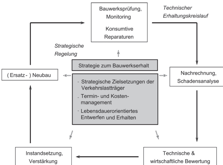
Bild 9. Kreislauf der Erhaltung und strategische Regelung (nach [17])
