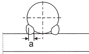
Bild 4.2. Wirksame Nahtdicke von Hohlkehlnähten an Vollquerschnitten
