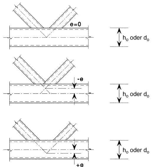
Bild 5.3. Knotenexzentrizitäten
