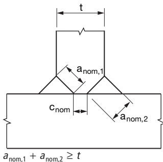
Bild 4.6. Wirksam durchgeschweißter T-Stoß
