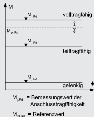
Bild K4. Anschlussklassifizierung nach der Beanspruchbarkeit
