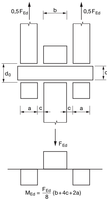
Bild 3.11. Biegemoment in einem Bolzen
