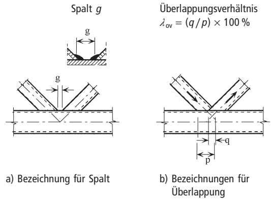
Bild 1.3. Knotenanschlüsse mit Spalt und mit Überlappung
