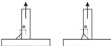
b) Zugkraft erzeugt Zug in der Schweißnahtwurzel
