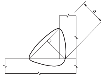
Bild 4.4. Kehl-nahtdicke bei tiefem Einbrand
