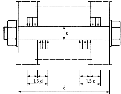
Bild 3.6. Begrenzung der effektiven Länge von langen Injektionsschrauben
