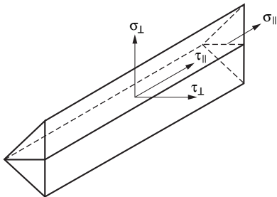
Bild 4.5. Spannungen im wirksamen Kehl-nahtquerschnitt
