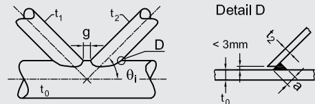
Bild K13. Knotenanschluss mit Spalt
