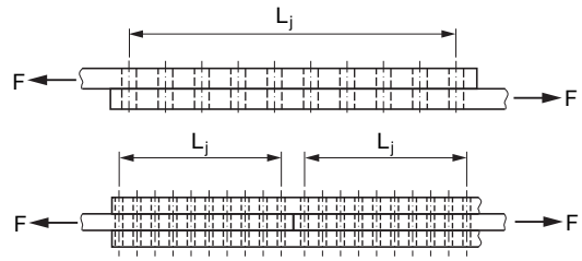
Bild 3.7. Lange Anschlüsse
