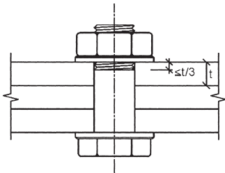
Bild 3.2. In ein Schraubenloch hineinragendes Gewinde von Passschrauben
