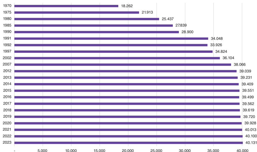
Abb. 1.2 Bestandsentwicklung der Bauwerke der Bundesfernstraßen; Stand 01.09.2023. Quelle: BASt.
