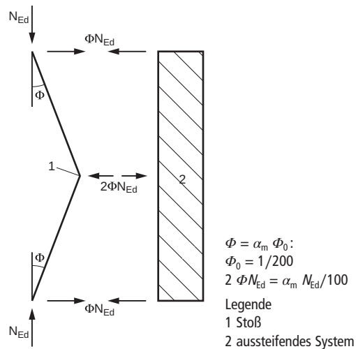
Bild 5.7. Lokale Ersatzkräfte an Stößen in druckbeanspruchten Bauteilen
