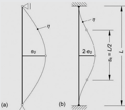
Bild K1. Ansatz der Imperfectionen bei einem gelenkig gelagerten Stab (a) und beidseitig eingespannten Stab (b) (nur qualitativer Vergleich)
