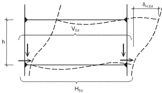
Bild 5.1. Bezeichnungen zu 5.2.1(4)
