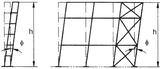
Bild 5.2. Äquivalente Stützenschiefstellung
