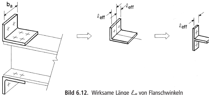
Bild 6.12. Wirksame Länge l_{eff} von Flanschwinkeln
