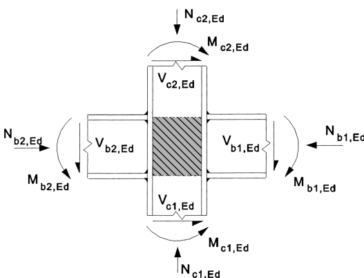
a) Werte am Schnitt des Stegfeldes
