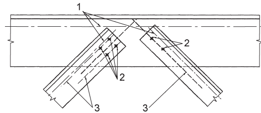
Legende 1 Schwerpunktsachsen 2 Verbindungsmittel 3 Bezugsachsen Bild 2.1. Bezugsachsen
