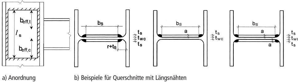
Bild 6.5. Beispiele für Verstärkungen mit zusätzlichen Stegblechen
