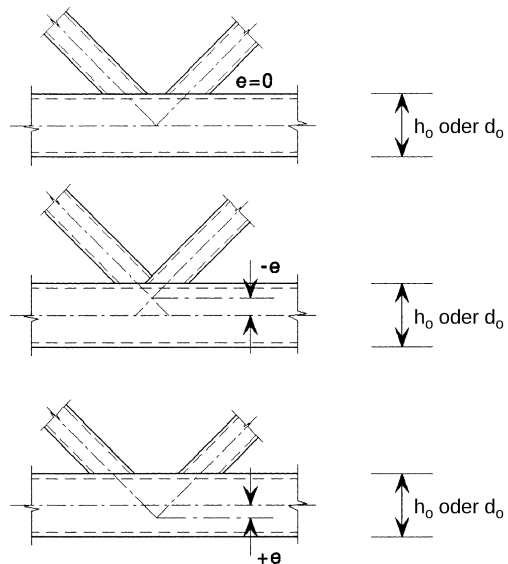
Bild 5.3. Knotenexzentrizitäten
