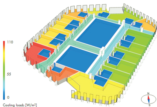
Bild 8 Wasl Tower, Dubai – Thermische Simulationen (WSGT)
