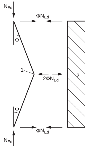
Bild 5.7. Lokale Ersatzkräfte an Stößen in druckbeanspruchten Bauteilen
