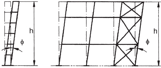
Bild 5.2. Äquivalente Stützenschiefstellung
