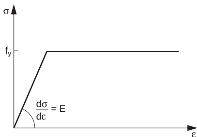
Bild 5.8. Bi-lineare Spannungs-Dehnungsbeziehung
