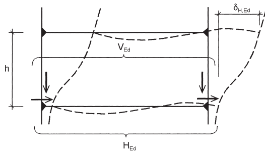
Bild 5.1. Bezeichnungen zu 5.2.1(4)
