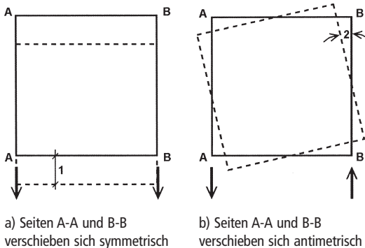
Bild 5.5. Verschiebungsmöglichkeiten und Einflüsse aus Torsion (Draufsicht)
