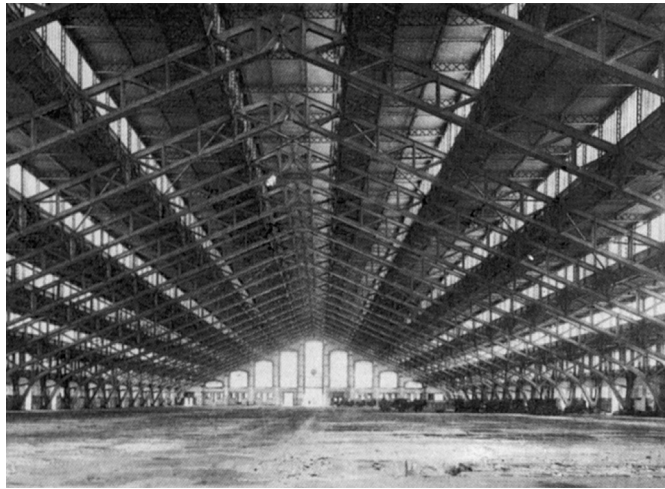
Bild 1.5 Schlachthöfe von Lyon, 1917. Foto: Inventaire général Rhône-Alpes, ADAGP, L.M. Raffle, 1997
