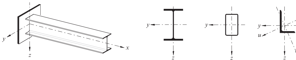
(a) Stabelement mit Koordinatensystem
