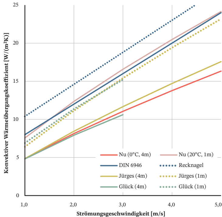
Bild 4. Resultierende Wärmeübergangskoeffizienten der unterschiedlichen Ansätze über die Nusselt-Zahl (Nu), die DIN EN ISO 6946 sowie über die vereinfachten Ansätze nach Recknagel , Jürges und Glück in Abhängigkeit der Strömungsgeschwindigkeit
