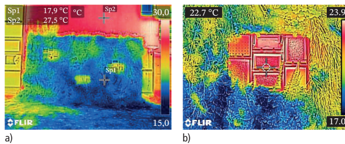
Bild 11. Thermographische Aufnahme der UNA-TERRA-Fassade in den Abendstunden nach einem strahlungsreichen Tag im Juli 2022; a) die gesamte Fassade, b) eine Detailaufnahme der Nisthilfe
