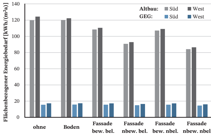
Bild 26. Auswirkungen der Fassadenbegrünung (Boden: bodengebunden System, Fassade: fassadenintegriertes System, (n)bew.: (nicht) bewässertes Substrat, (n)bel.: (nicht) hinterlüftet) auf den flächenbezogenen Energiebedarf der untersuchten Räume. Als Referenz sind die Werte ohne Begrünung dargestellt.
