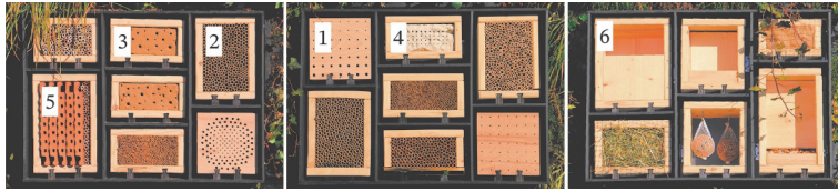
Bild 6. Fotografische Aufnahme der unterschiedlichen verbauten Nisthilfesysteme an der UNA-TERRA-Fassade auf dem Campus Vaihingen der Universität Stuttgart
