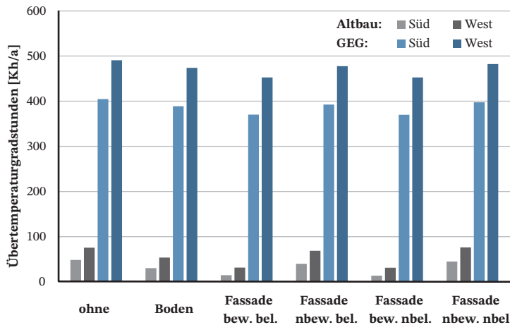
Bild 27. Auswirkungen der Fassadenbegrünung (Boden: bodengebunden System, Fassade: fassadenintegriertes System, (n)bew.: (nicht) bewässertes Substrat, (n)bel.: (nicht) hinterlüftet) auf den sommerlichen Wärmeschutz anhand der Übertemperaturgradstunden der untersuchten Räume. Als Referenz sind die Werte ohne Begrünung dargestellt.
