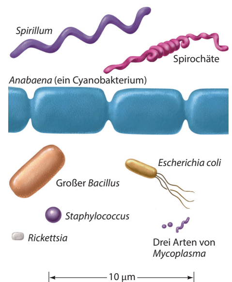
Abb. 1.7 Maßstabgerechte Darstellung verschiedener prokaryotischer Zellen.
