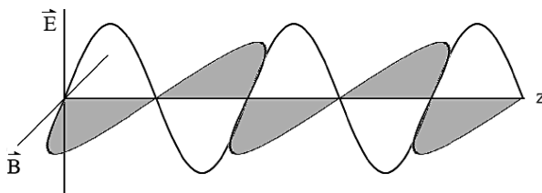
Abb. 1.1 Beschreibung der Ausbreitung einer linear polarisierten elektromagnetischen Welle als Schwingung des elektrischen ( \vec{E} ) und magnetischen ( \vec{B} ) Felds.
