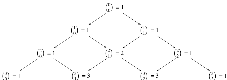
Abb. 1.2 Pascal'sches Dreieck.
