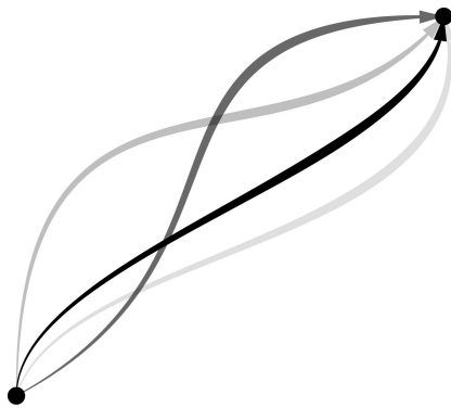
Abb. 1.3 Die lagrangesche Formulierung der Mechanik betrachtet alle möglichen Wege von einem Start- zu einem Endpunkt. Der tatsächliche Weg – der Weg, den ein Teilchen natürlicherweise nehmen würde – ist derjenige, für den eine als Wirkung bezeichnete Größe minimal ist.
