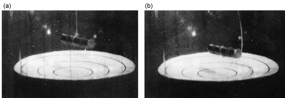
Abb. 1.5 Der »schwebende Magnet« zur Demonstration der Dauerströme in supraleitendem Blei, die beim Absenken durch Induktion angeworfen werden. (a) Ausgangslage, (b) Gleichgewichtslage.
