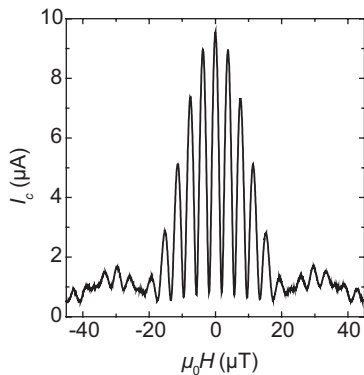
Abb. 1.30 Magnetfeldabhängigkeit des maximalen Suprastroms einer SQUID-Struktur aus \text{YBa}_2\text{Cu}_3\text{O}_7 . Die beiden Josephson-Kontakte sind 9\ \mu\text{m} breit, so dass die I_c -Modulation der Einzelkontakte als Einhüllende der SQUID-Oszillationen sichtbar wird. Nach [49]. Ich danke C. Schneider und J. Mannhart für die Bereitstellung der Originaldaten.
