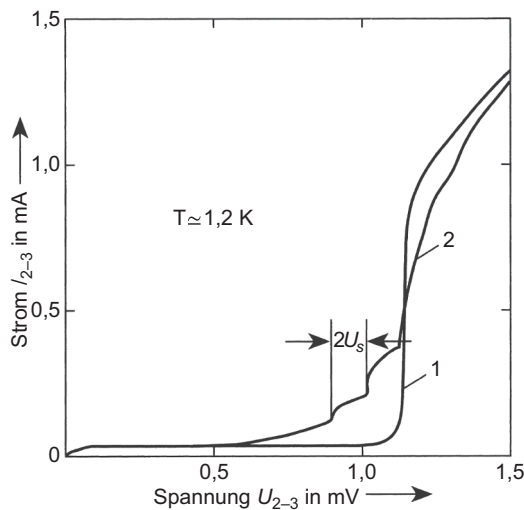
Abb. 1.24 Kennlinie des Kontaktes 2–3 aus Abb. 1.23. Kurve 1 ohne Spannung an Kontakt 1–2, Kurve 2 mit 0,055 mV an Kontakt 1–2. Nach [42]; © 1965 American Physical Society.
