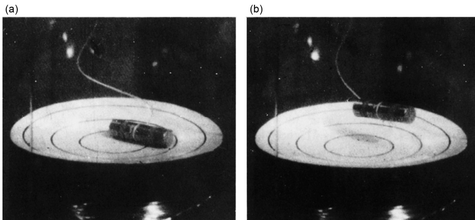
Abb. 1.7 »Schwebender Magnet« zur Demonstration des Meißner-Ochsenfeld-Effekts bei angelegtem Magnetfeld. (a) Ausgangslage für T > T_c , (b) Gleichgewichtslage für T < T_c .
