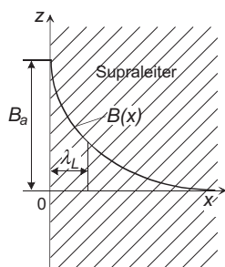
Abb. 1.15 Abnahme des magnetischen Felds im Supraleiter nahe einer ebenen Oberfläche.
