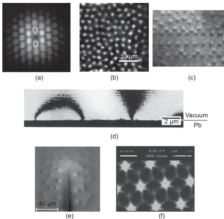
Abb. 1.10 Methoden zur Abbildung von Flussschläuchen: (a) Neutronen-Beugungsbild des Vortextgitters in Niob; (b) Magnetooptische Abbildung von Flusswirbeln in \text{NbSe}_2 [10]; (c) Lorentz-Mikroskopie an Niob; (d) Elektronenholographie an Pb [12], (e) Tieftemperatur-Rasterelektronenmikroskopie an \text{YBa}_2\text{Cu}_3\text{O}_7 [15] (f) Rastertunnelmikroskopie an \text{NbSe}_2 . Abb. (a) mit freundlicher Genehmigung durch das Institut Max von Laue-Paul Langevin, Grenoble [9]. Abb. (b) mit Erlaubnis von [10]; © IOP Publishing 2001. All rights reserved. Abb. (c) mit freundlicher Genehmigung durch A. Tonomura, Fa. Hitachi Ltd., 2003. Abb. (d) mit Erlaubnis von [12], © 1989 American Physical Society. Abb. (e) mit Erlaubnis von [14], © 2004 AIP Publishing; Abb. (f) mit freundlicher Genehmigung durch Fa. Lucent Technologies Inc./Bell Labs (2003).
