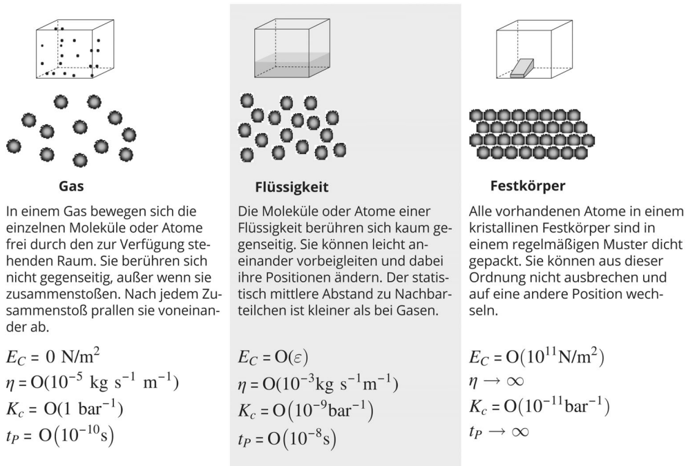
Abbildung 1.1: Vergleich der Eigenschaften von Gasen, Flüssigkeiten und Festkörpern. E_C = Elastizitätsmodul in N/m 2 , \eta = Viskosität in kg/(m s), K_C = Kompressibilität in bar -1 , t_P = Platzwechselzeiten der Teilchen in Sekunden, O(\varepsilon) = Ordnung \varepsilon , mit \varepsilon > 0 und \varepsilon \ll 1
