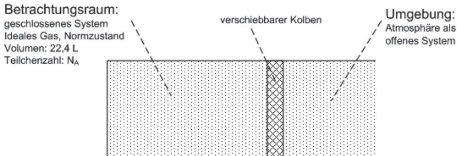
Abbildung 1.1: Ideales Gas in einem geschlossenen System
