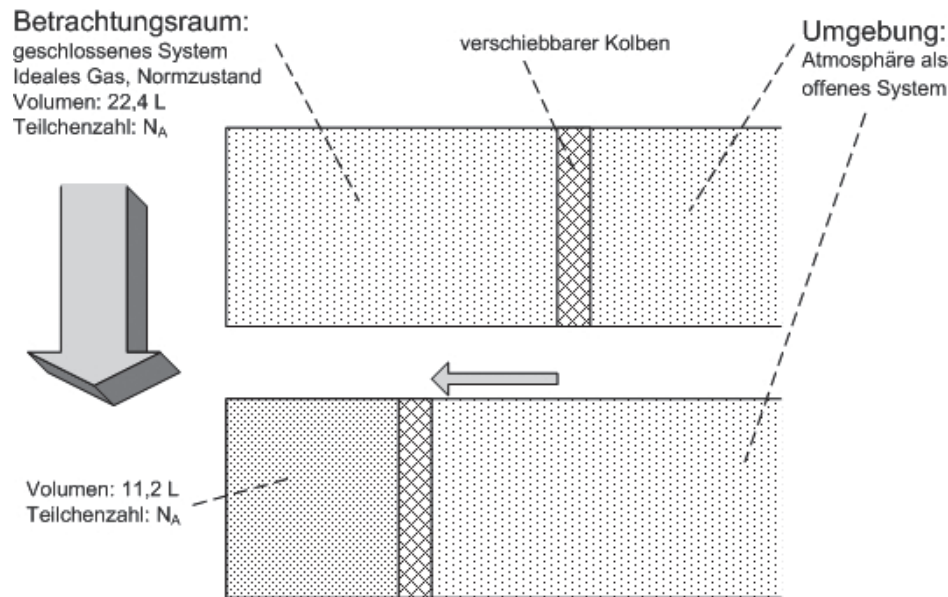
Abbildung 1.2: Druckerhöhung durch Volumenverkleinerung
