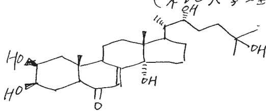
d-Ecdysone
