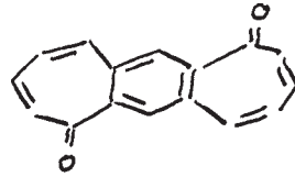
Ditylro tropacenedione
