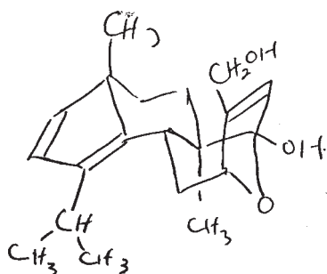
allocyathin B 3 .
