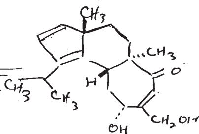
allocyathin B 3 .
