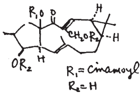
Jolkinol A
