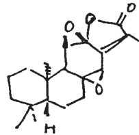
Jolkinolide B
