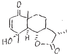
Vulagarin
