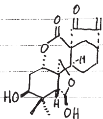
enmein
