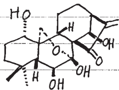
oridonin
